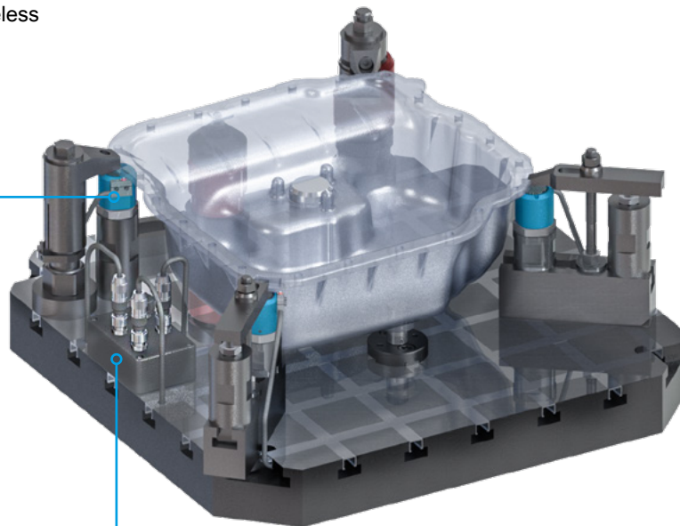
Transmițător wireless
