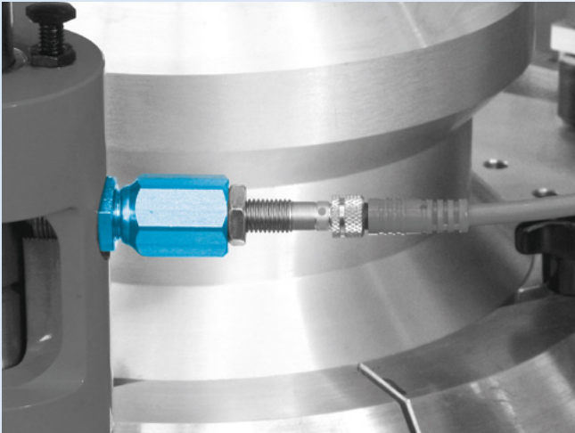
Sensor elementen voor positiebepaling met behulp van inductieve standaardensoren. Afgebeeld is de compacte uitvoering met fijne schroefdraad.
