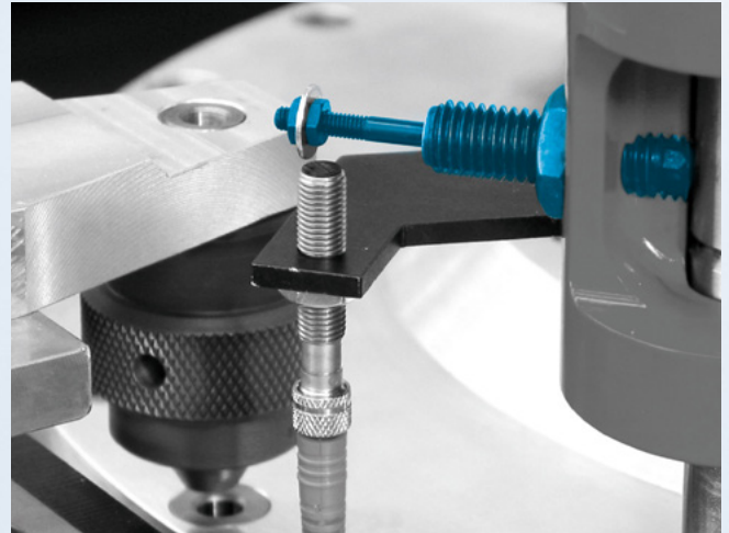
Er zijn ook uitvoeringen leverbaar met een tegen verdraaien geborgde schakelpen.
