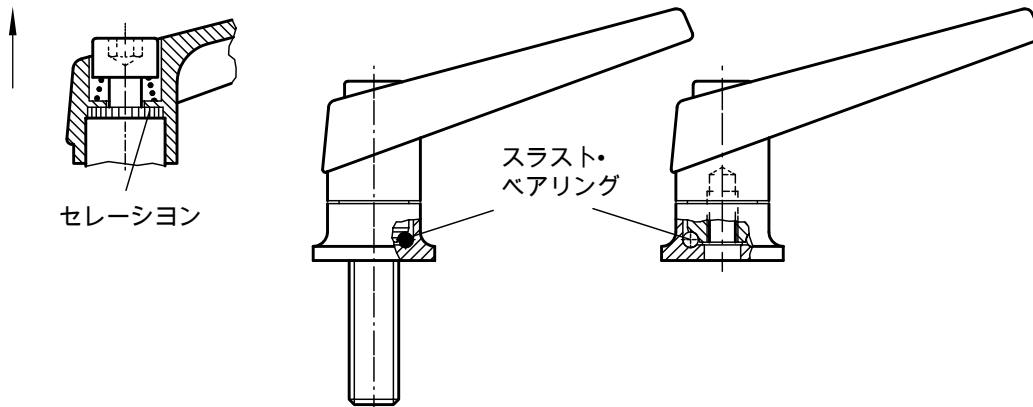
スラスト・ベアリングによるクランプ力の向上 (手で同じ力を加えた場合)
