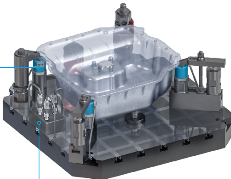
Trasmittitore wireless
