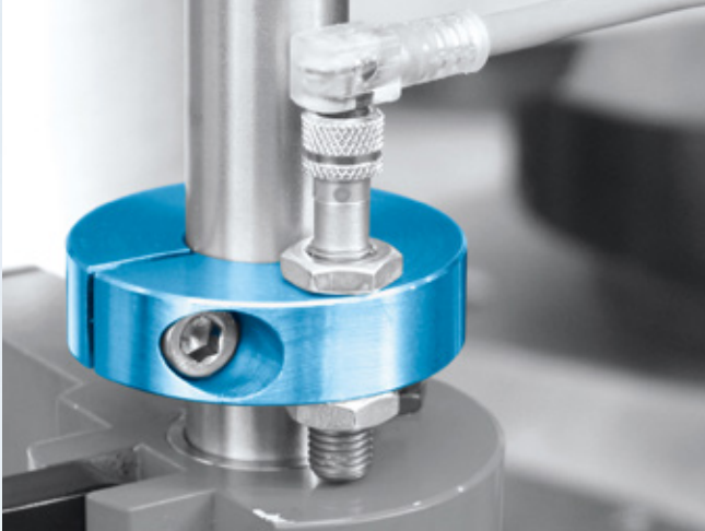
Asetinrenkaat ovat yleiskäyttöisiä, esim. kiinteänä vasteena. Kuvassa malli, jossa sensoriadapteri.
