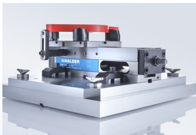
Příklad použití EH 23111. Upínací čepý pro rychlou výměnu na stole stroje.
