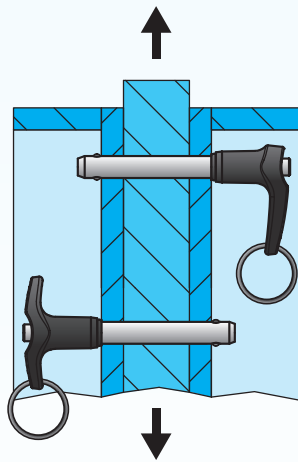
Scherbelastung zweischnittig
